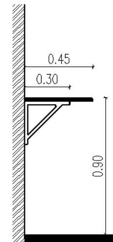
Mesa de Apoyo con ménsula
